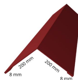
Hófogó
