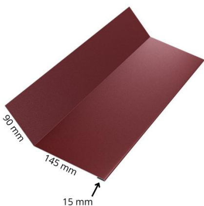
Törésvonalszegély
